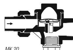
MK 20
