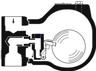
UNA 14 P
