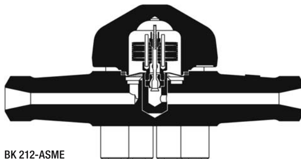
BK 212-ASME
