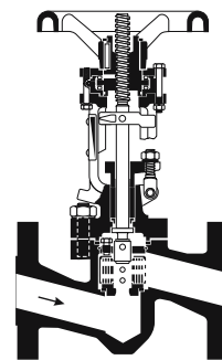
ZK 29
