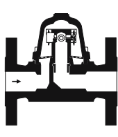
MK 25/2 DN 40/50
