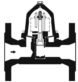
BK 27 N
